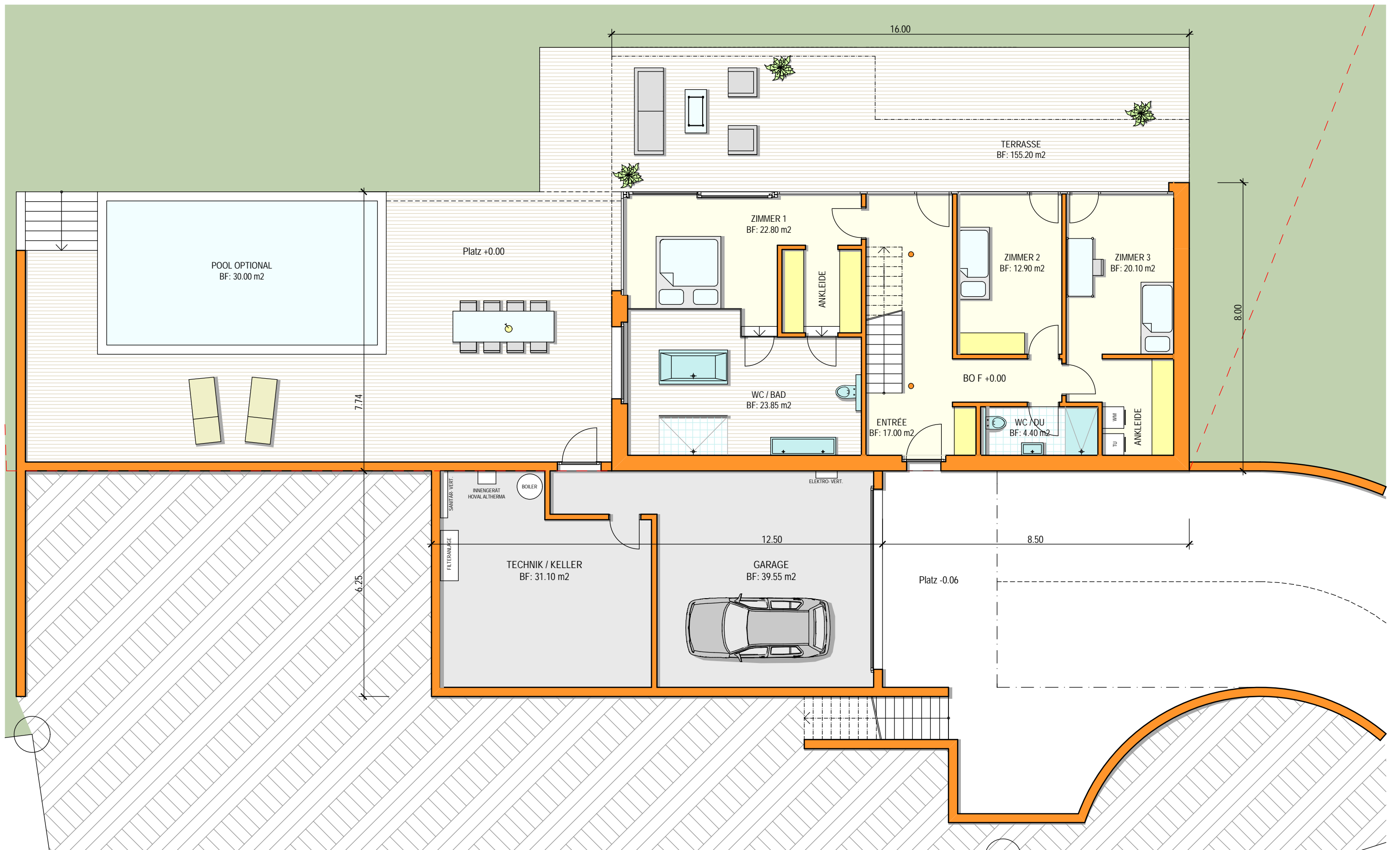
GRUNDRISS ERDGESCHOSS 1:100
